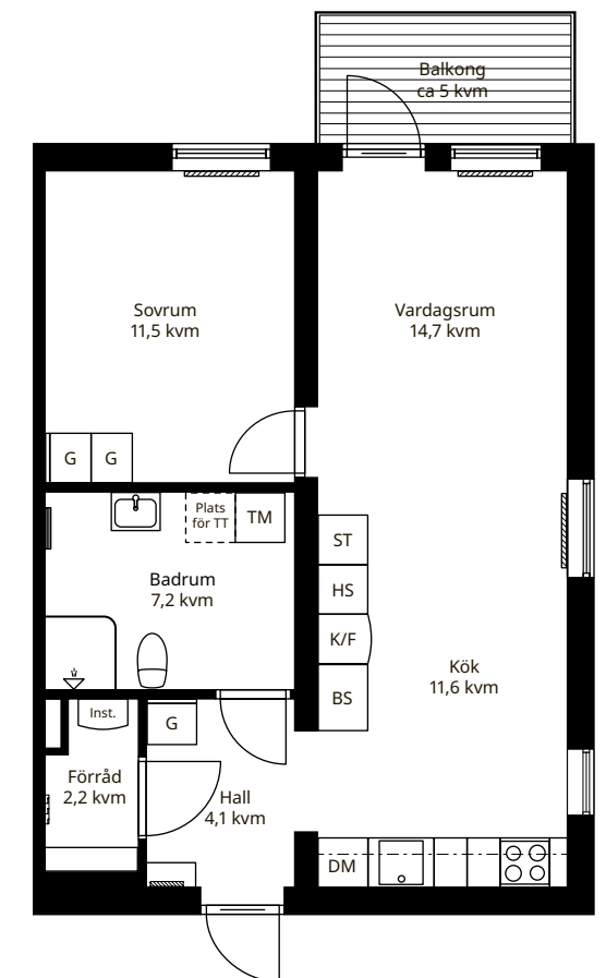
Rätvänd planlösning, gavel, skala 1:100
